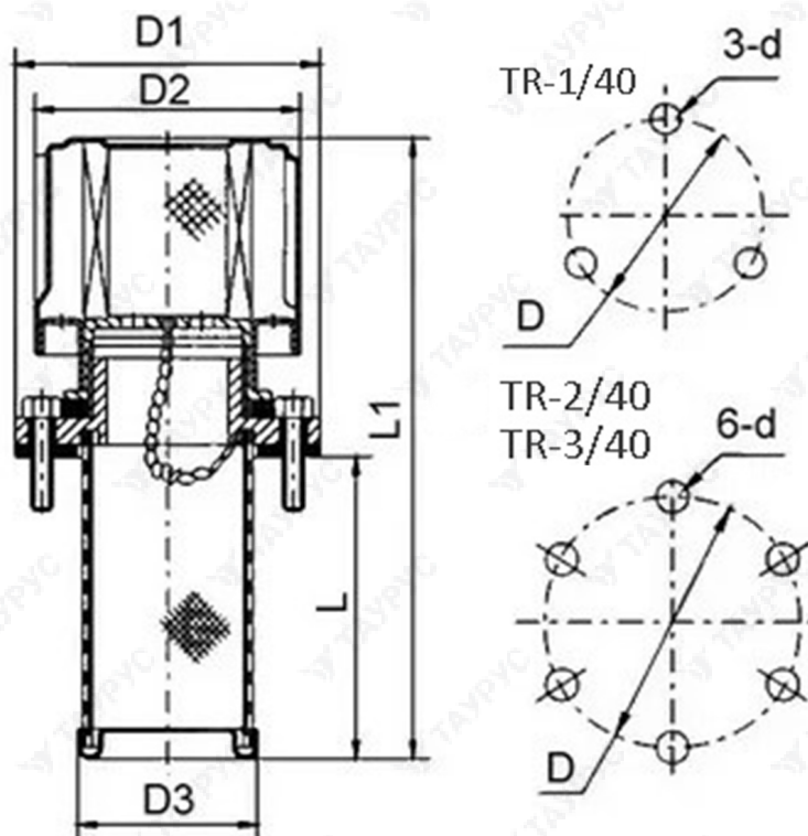
Чертеж заливной горловины TR-x/40
