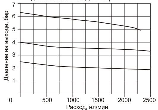
Регулировочные характеристики
