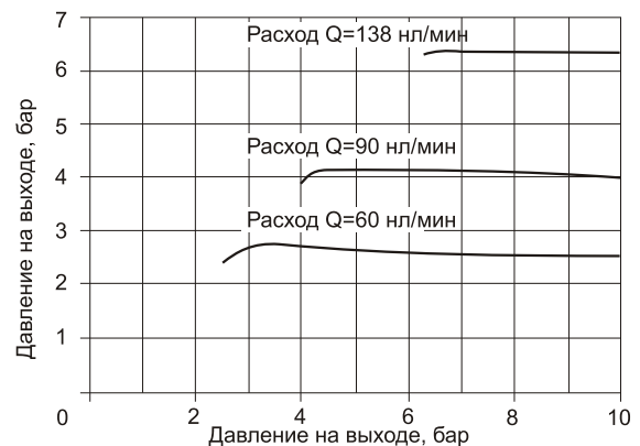
Регулировочные характеристики
