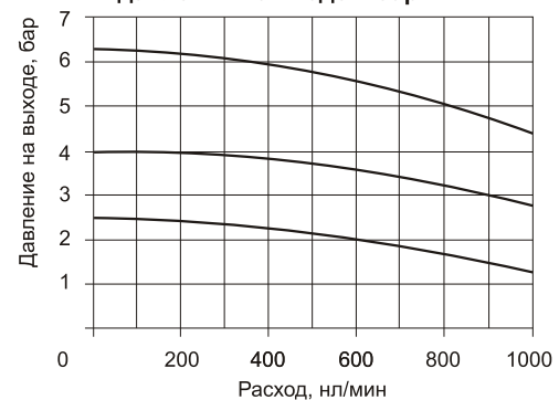
Регулировочные характеристики
