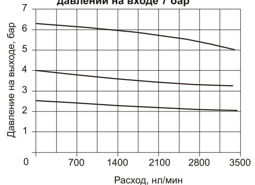
Регулировочные характеристики
