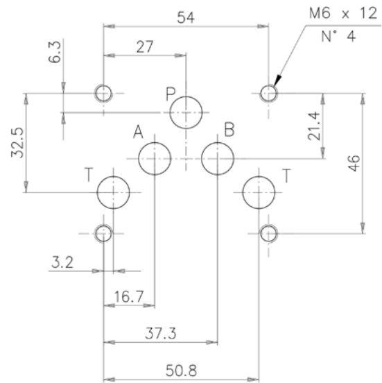
СЕТОР 5 Ду10
