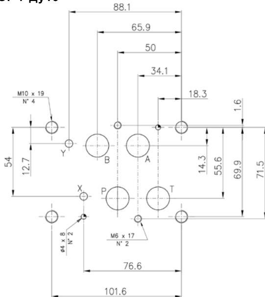
СЕТОР 7 Ду16
