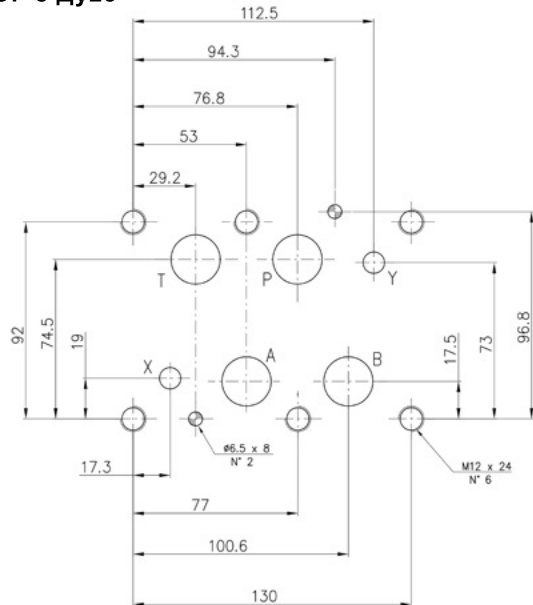
СЕТОР 8 Ду25
